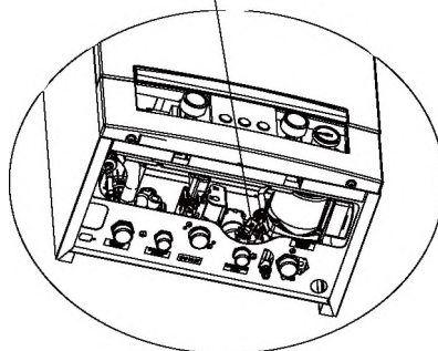
Кран заполнения системы отопления
